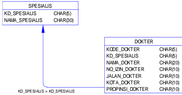
Gambar 2. ERD PDM Relasi Dokter dan Spesialis
