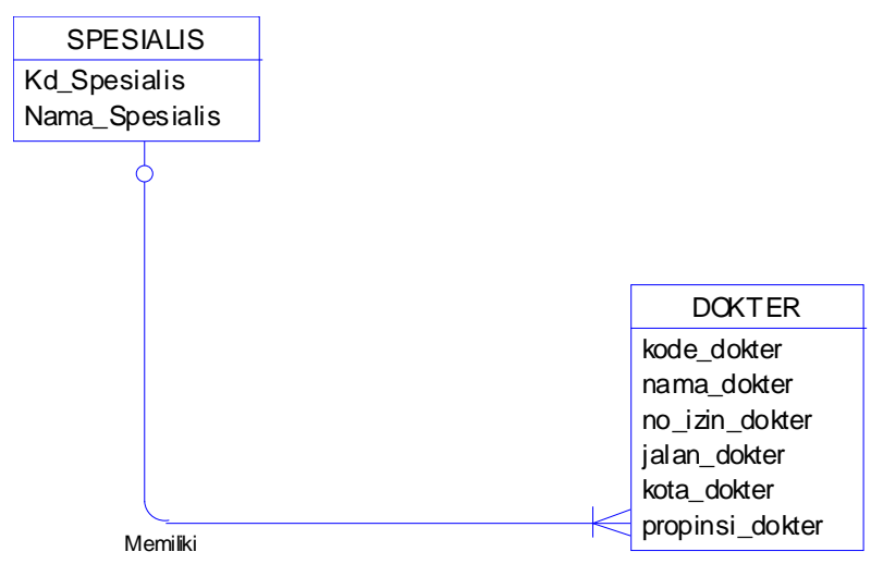
Gambar 1. ERD CDM Relasi Dokter dan Spesialis
