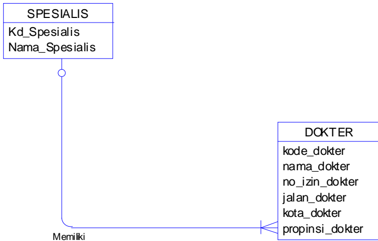
Gambar 1. ERD CDM Relasi Dokter dan Spesialis
