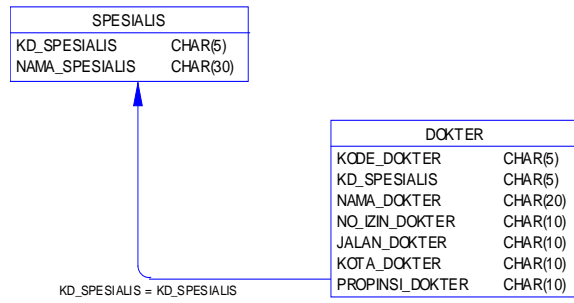
Gambar 2. ERD PDM Relasi Dokter dan Spesialis
